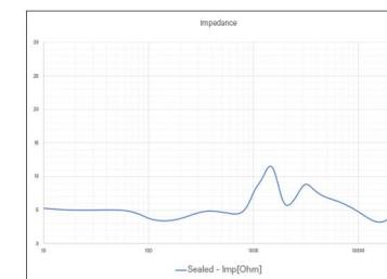
阻抗
