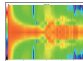
垂直指向性
