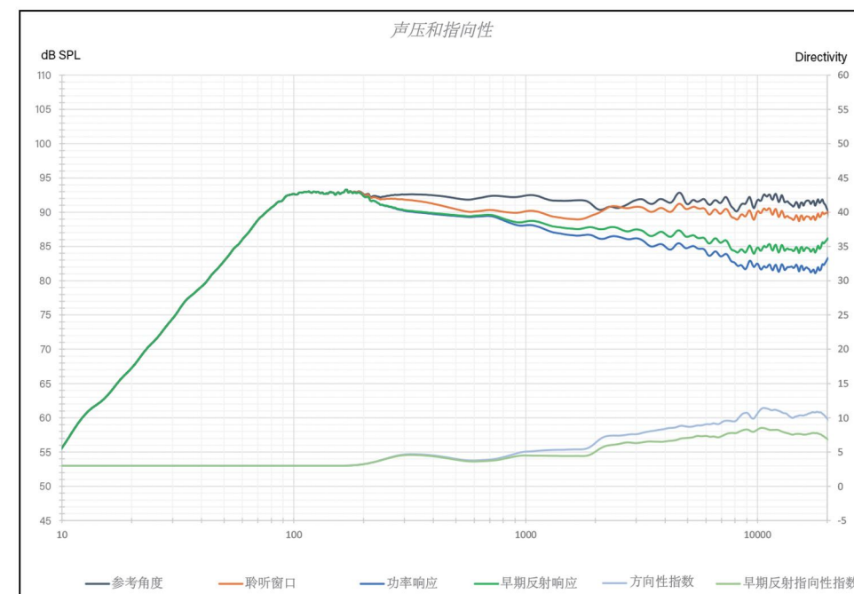
水平指向性
