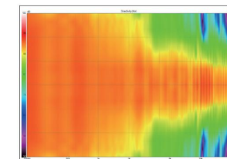
垂直指向性
