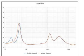
阻抗
