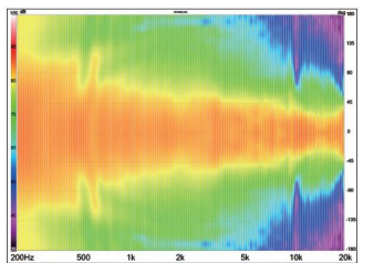
垂直指向性
