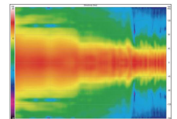
垂直指向性
